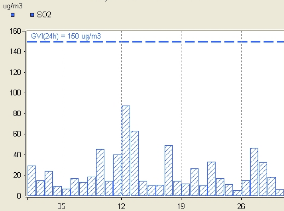
Voljovica SO2 1.4.2009 - 30.4.2009
