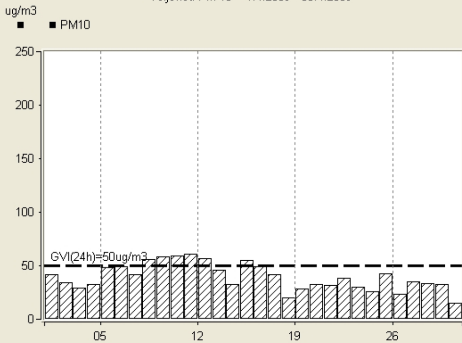
Voljovica PM 10 1.4.2009 - 30.4.2009
